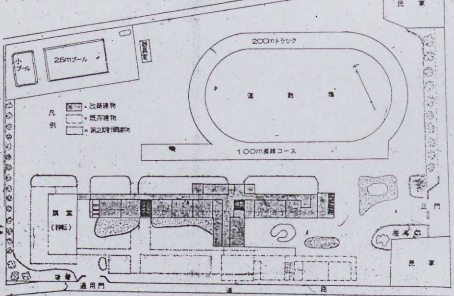
東益津小学校校舎改築計画平面図
