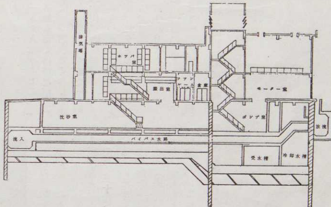
【新屋ポンプ場の断面図】
